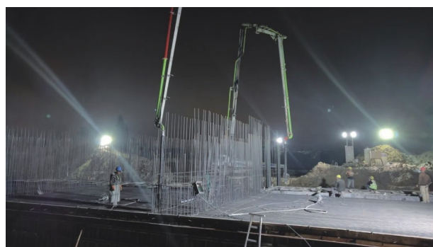
云霄县北江水闸底板首次浇筑现场
