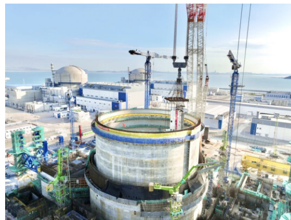
环路蒸发器隔间混凝土模块吊装中
